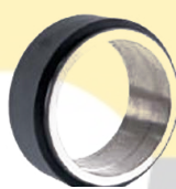
LGV Drive Wheel(PPDI) D230xW80(STEEL CORE)
